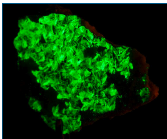
Figura 1. Imagen de un ejemplar del mineral "autunita", fosfato uranílico hidratado [\text{Ca}(\text{UO}_2)_2(\text{PO}_4)_2 \cdot 10\text{--}12\text{H}_2\text{O}] fotografiado bajo luz ultravioleta [6]
